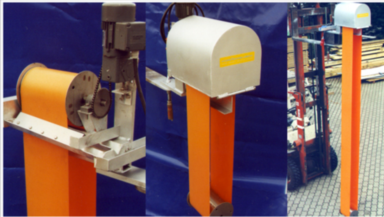
Bandskimmer
