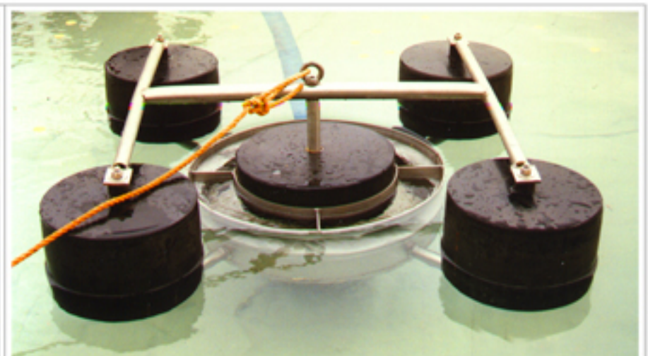
Trogskimmer MAXI 4
